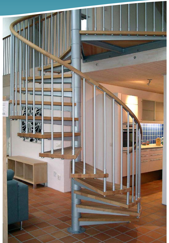
Floby typ Lövdalen med barnsäkert räcke.
